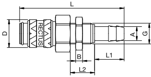
Schottverschraubung für Schlauchanschluss
