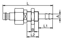
Schottverschraubung für Schlauchanschluss
