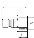
Innengewinde
